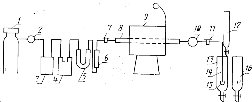
Схема установки для определения серы титриметрическим методом
